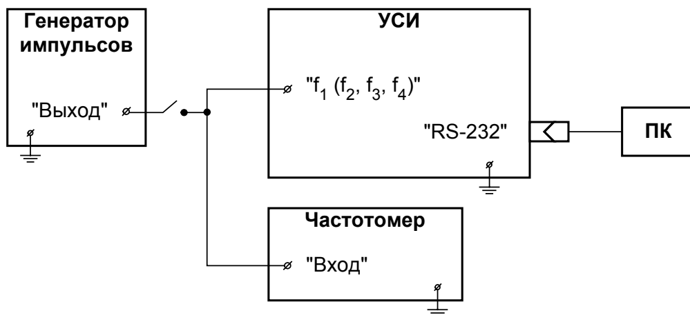
Рис. 26. Схема подключения модуля счетчика импульсов при поверке.
