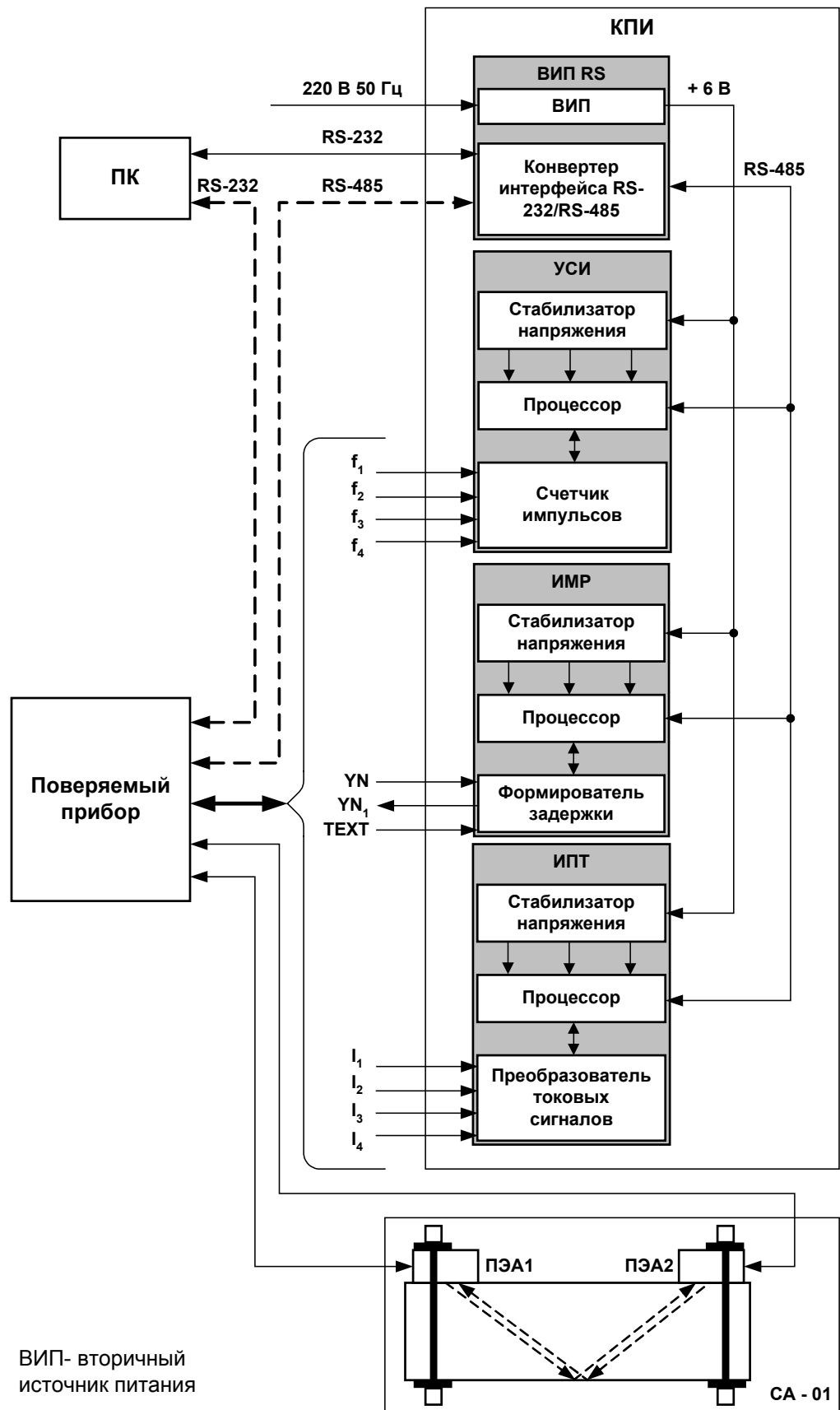
Рис. 1. Структурная схема КПИВ-010.
