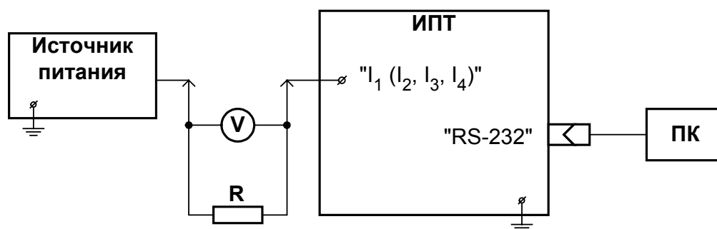
Рис. 28. Схема подключения модуля измерителя постоянного тока при поверке.
